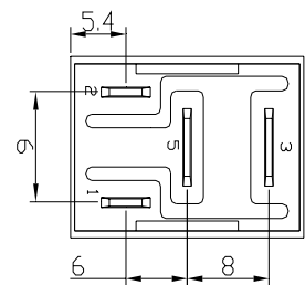
A 型接线图
