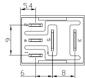
C 型接线图
