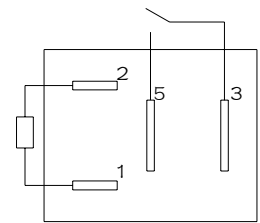
A 型接线图
