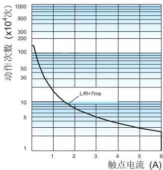
直流感性负载电耐久性曲线
