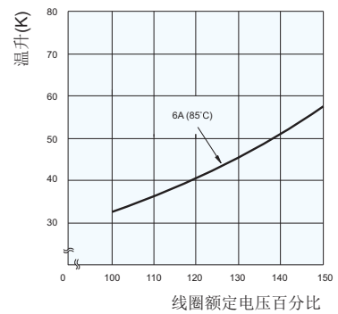
线圈温升
