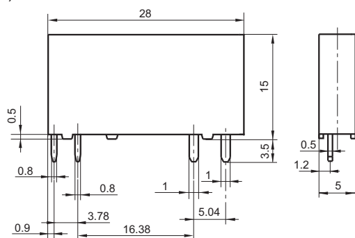
外形图
